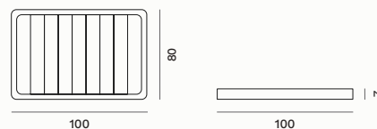
Shower tray / Piatto doccia / Receveur de douche PIADOFUN
