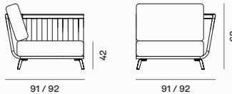
Lt module / Modulo sx / Module g
