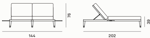
Double sunlounger / Lettino doppio / Bain de soleil double
