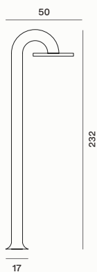
Solar Shower / Doccia solare / Douche solaire DOFUN
