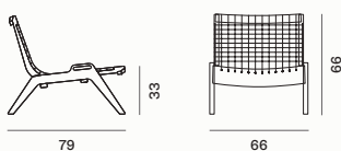
Lounge armchair stackable / Poltrona lounge impilabile / Fauteuil lounge empilable POLOS
