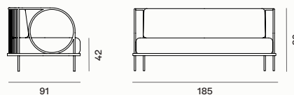
Sofa / Divano / Canapé ARIDIVGBR
