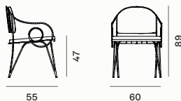
Small armchair / Poltroncina / Petit fauteuil ARIPOBR
