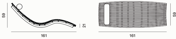
Sunlounger / Lettino / Bain de soleil SWIDO
