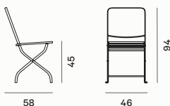
Chair / Sedia / Chaise CESEG
