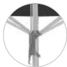
Une ouverture et une fermeture rapides avec coulisse et levier de serrage sont possibles grâce au principe télescopique.
