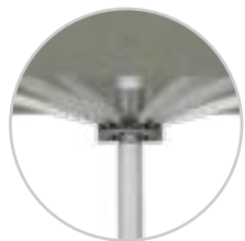
La structure est en profilés d'aluminium extrudé (pressé, anodisé naturel) avec mât antidéformation (nervures de renfort incl.).
